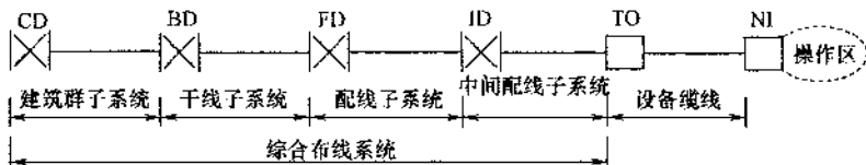
图 3.7.3 工业环境布线系统架构
