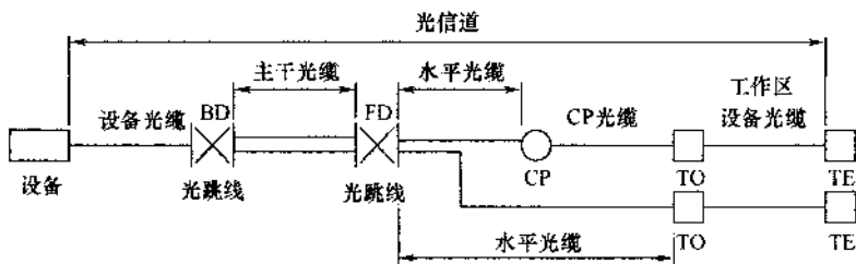
图 3.2.4-1 光纤信道构成 1
