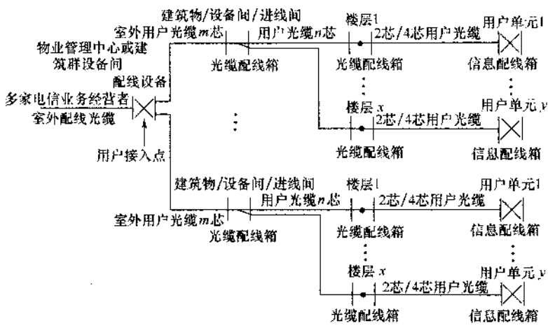
图 4.2.2-3 用户接入点设于建筑群物业管理中心机房或综合布线设备间或通信机房
