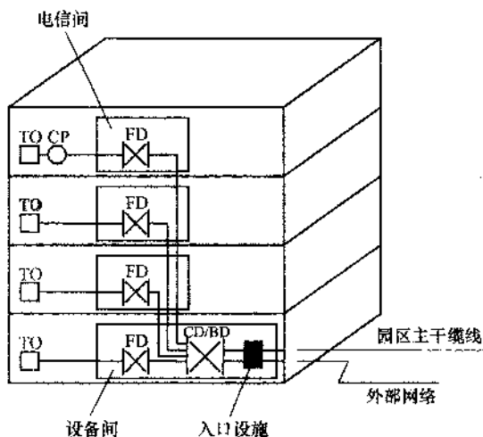
图1 综合布线配线设备典型设置
