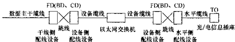
图 5.2.3-2 交叉连接方式
