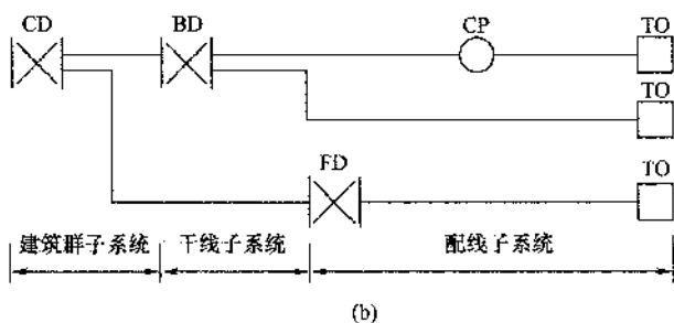
图 3.1.2-2 综合布线子系统构成
